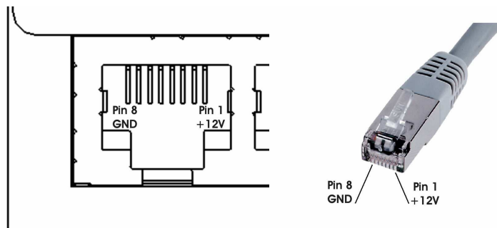
Pinbelegung RJ-45 Buchse
